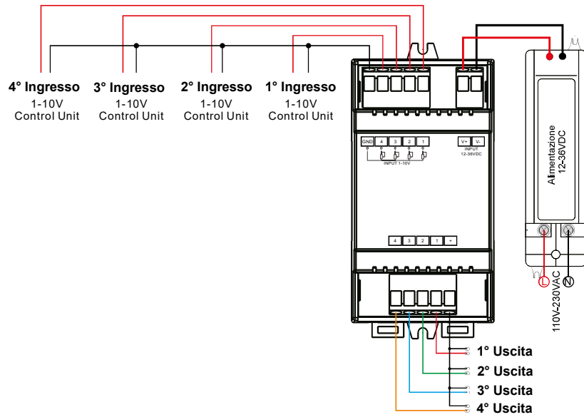
SCHEMA DI COLLEGAMENTO DIMMER STRIP LED codice TE110RGBW
